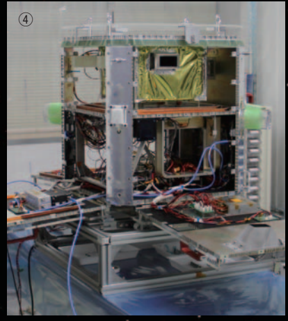
写真3 埃を防ぐクリーンルーム内で組立中のNano-JASMINE。
