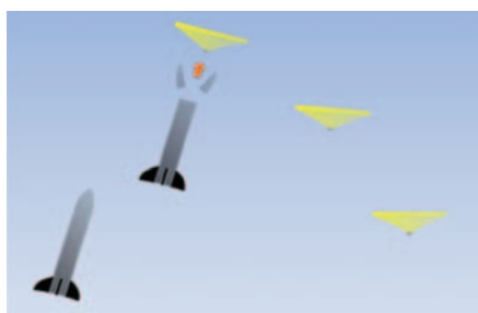
観測ロケットによる実験の様子。ロケットは上空で MAAC を放出、燃えずに地上まで降りてくる。
